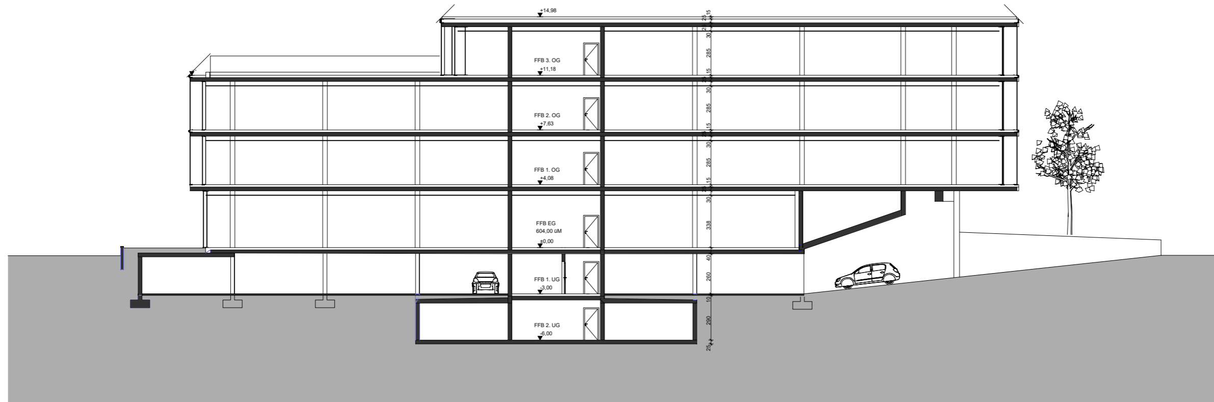
SCHNITT 02
